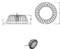
Technische Daten Osram PrevaLED Coin MR16 G2 12W 1200lm 40D - 830
